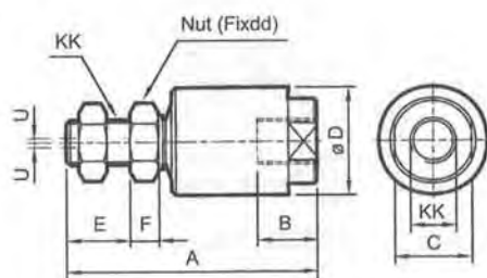
尺寸[mm]
