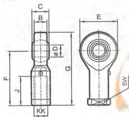
尺寸[mm]
